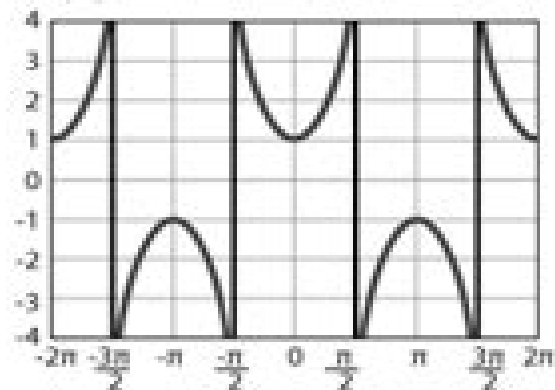
\sec(x)
