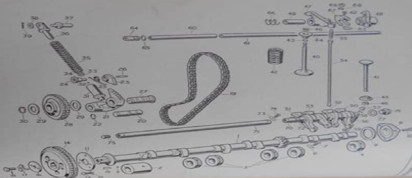
Fig. A-1. Valve gear.
