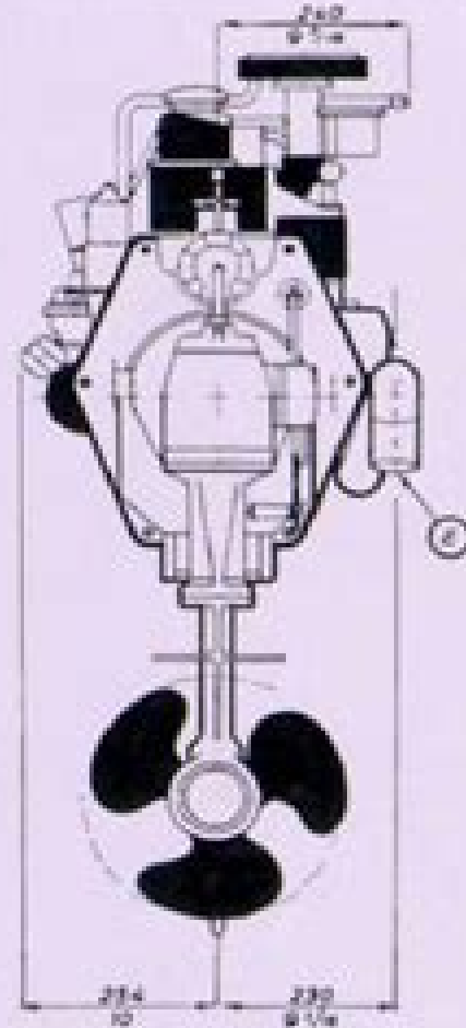
Volvo Penta AQ110 / 100
