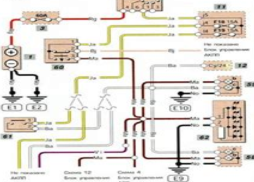
1. Схема 5. Аккумулятор включен, передний прожекторный фары
