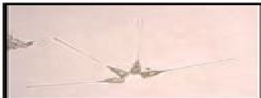
Asterionella
