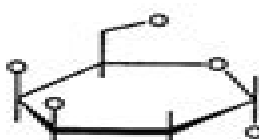
Galactose
