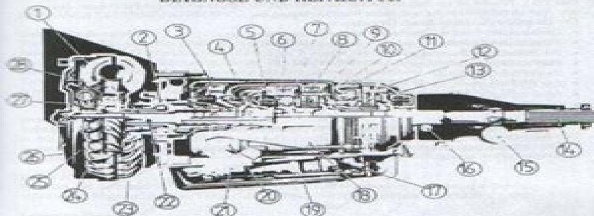
Bild 1 - TH 700-R4 Getriebe
