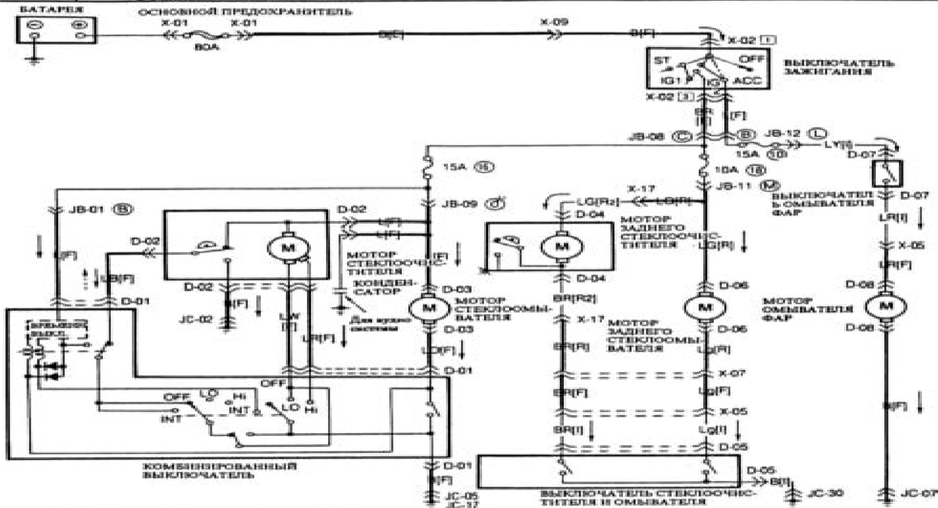
D-01 Комбинированный выкл.
