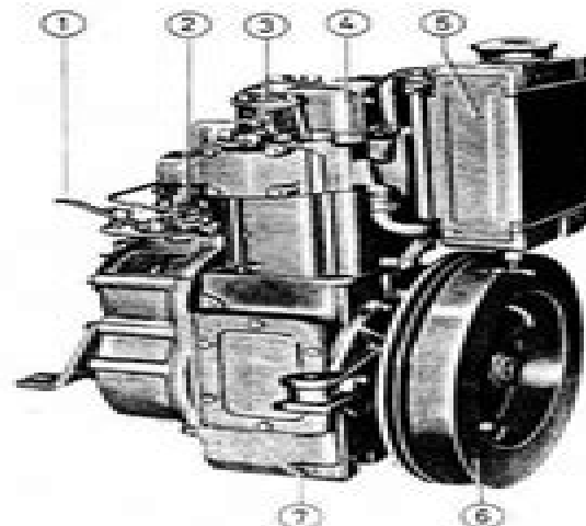
Fig 2. D1 engine
