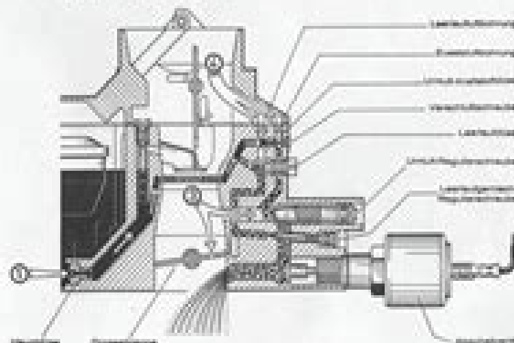
Bild 10: 34 PICT-3 Wirkungsweise des Leerlauf- und Umluftsystems ① = Zufuß des Kraftstoffes ② = Eintritt der Ausgleichluft ③ = Eintritt der Leerlaufuft
