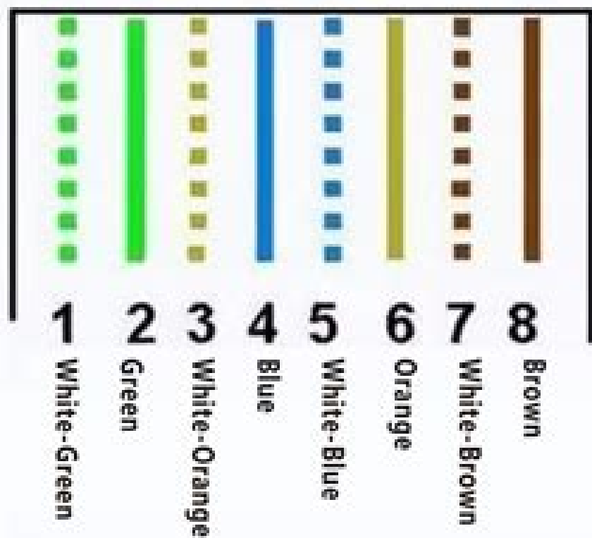
T568A
