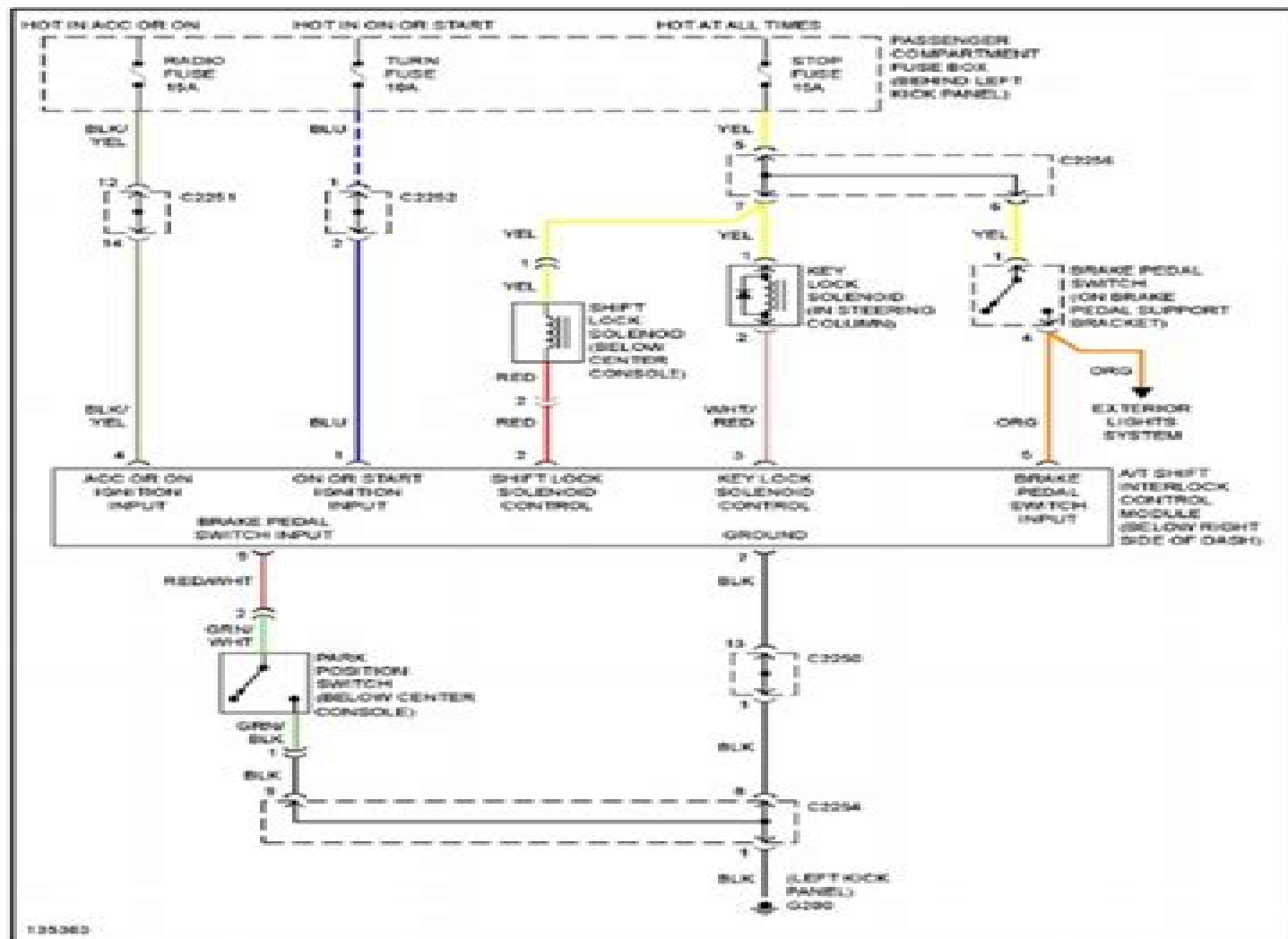
Fig. 34: Shift Interlock Circuit
